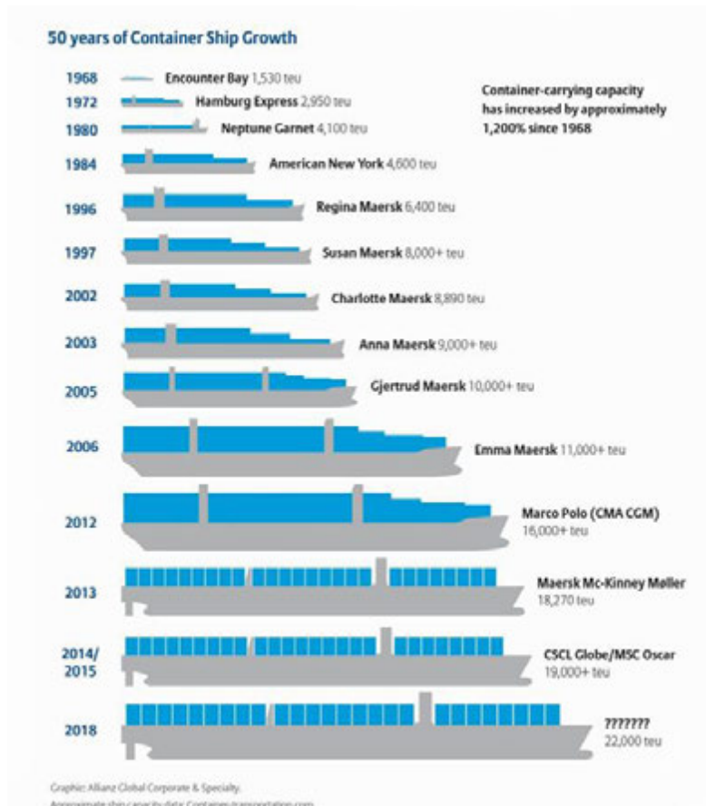
Figura 11: Evolución del Buque Portacontenedores en los últimos 50 años
